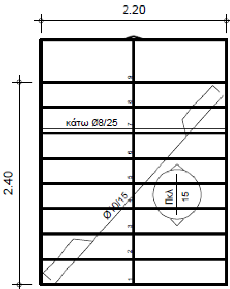
Σχήμα 1: Οπλισμός κλίμακας
