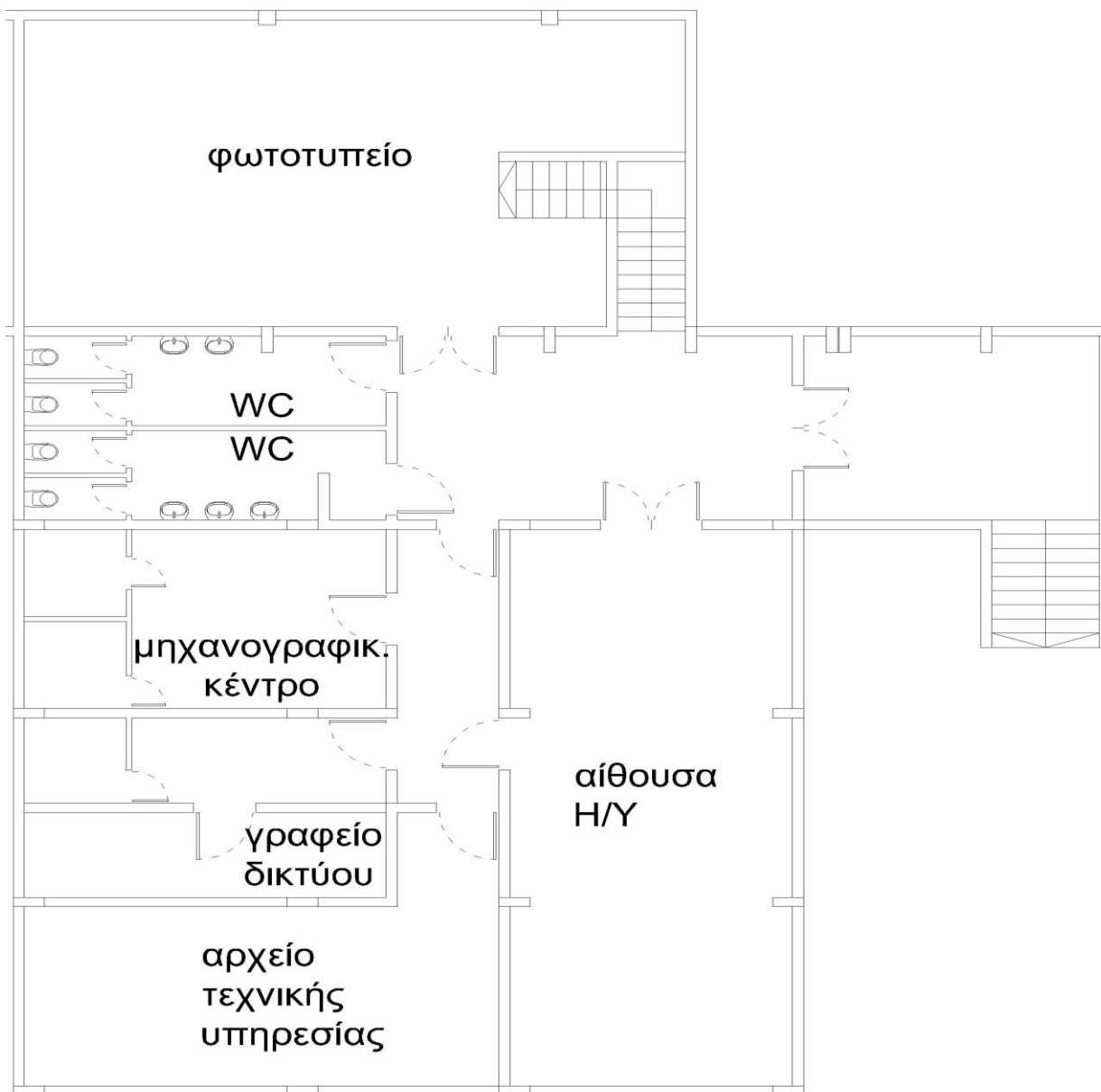
σχέδιο 1δ / κάτοψη υπογείου κλίμακα 1:100
