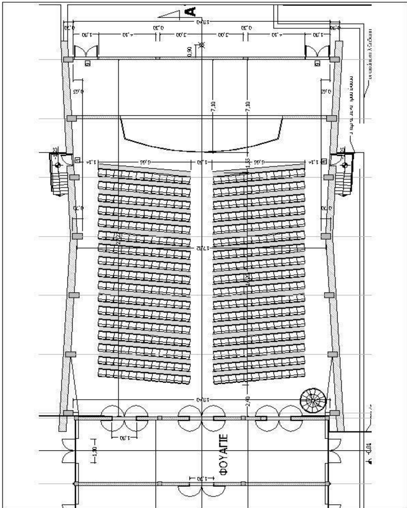
ΣΧΕΔΙΟ 2α: ΚΑΤΟΨΗ ΑΜΦΙΘΕΑΤΡΟΥ
